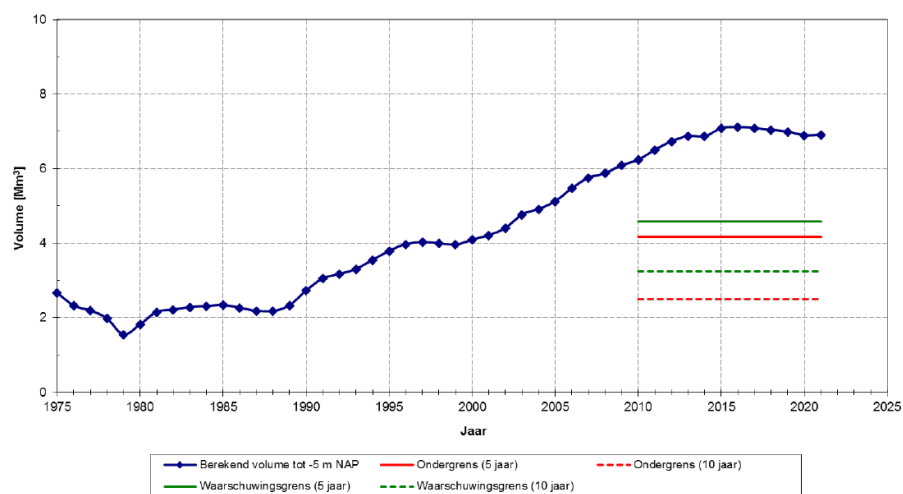
Macrocel 6 (Hoofdgeul)
