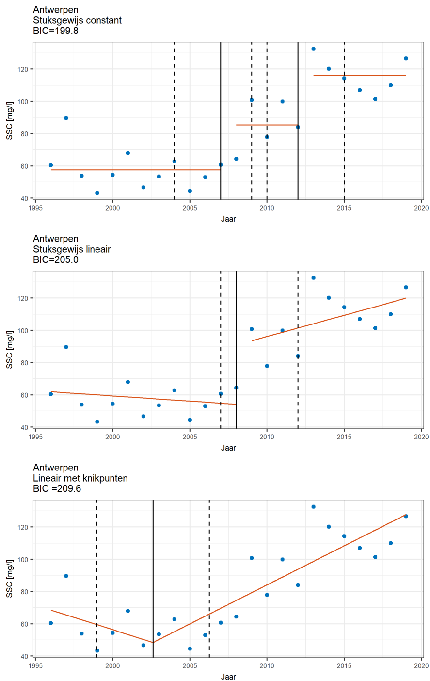
Bijlage - Figuur J-9: Drie verschillende types stuksgewijze regressie, gefit op de tijdreeks van sedimentconcentratie op meetlocatie Antwerpen. Verticale volle lijn geeft de geschatte locatie weer van de trendbreuk; verticale stippellijnen geven de 95%-betrouwbaarheidsintervallen weer.
