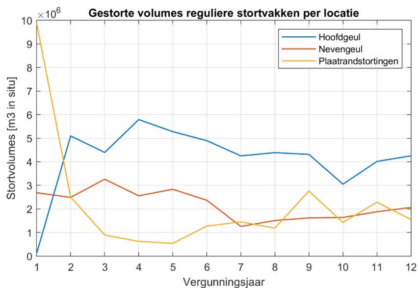
Bijlage - Figuur B-3: Stortvolume per vergunningsjaar per type stortlocatie, voor de reguliere stortvakken.
