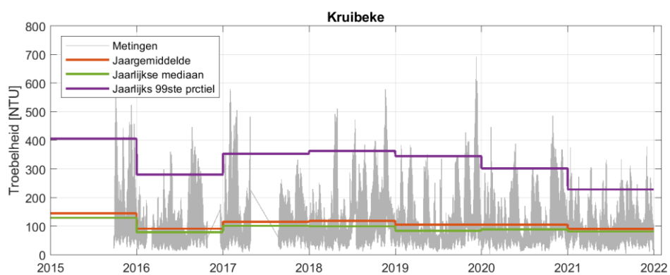
Bijlage - Figuur J-6: Continue metingen troebelheid Kruibeke.
