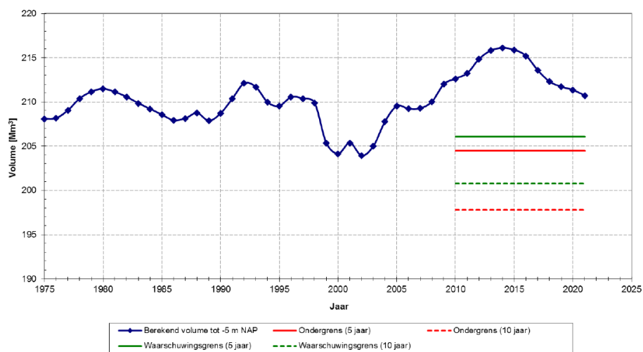
Macrocel 3 (Hoofdgeul)
