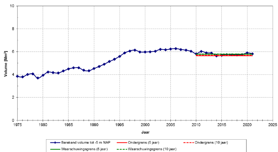
Macrocel 7 (Hoofdgeul)
