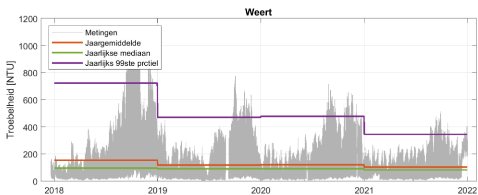
Bijlage - Figuur J-5: Continue metingen troebelheid Weert.
