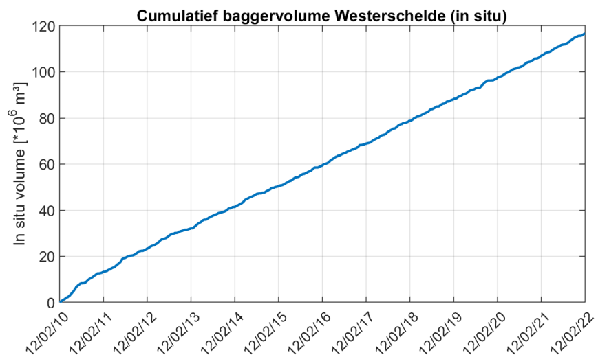
Bijlage - Figuur B-4: Cumulatief baggervolume volledige Westerschelde (in situ m 3 ).
