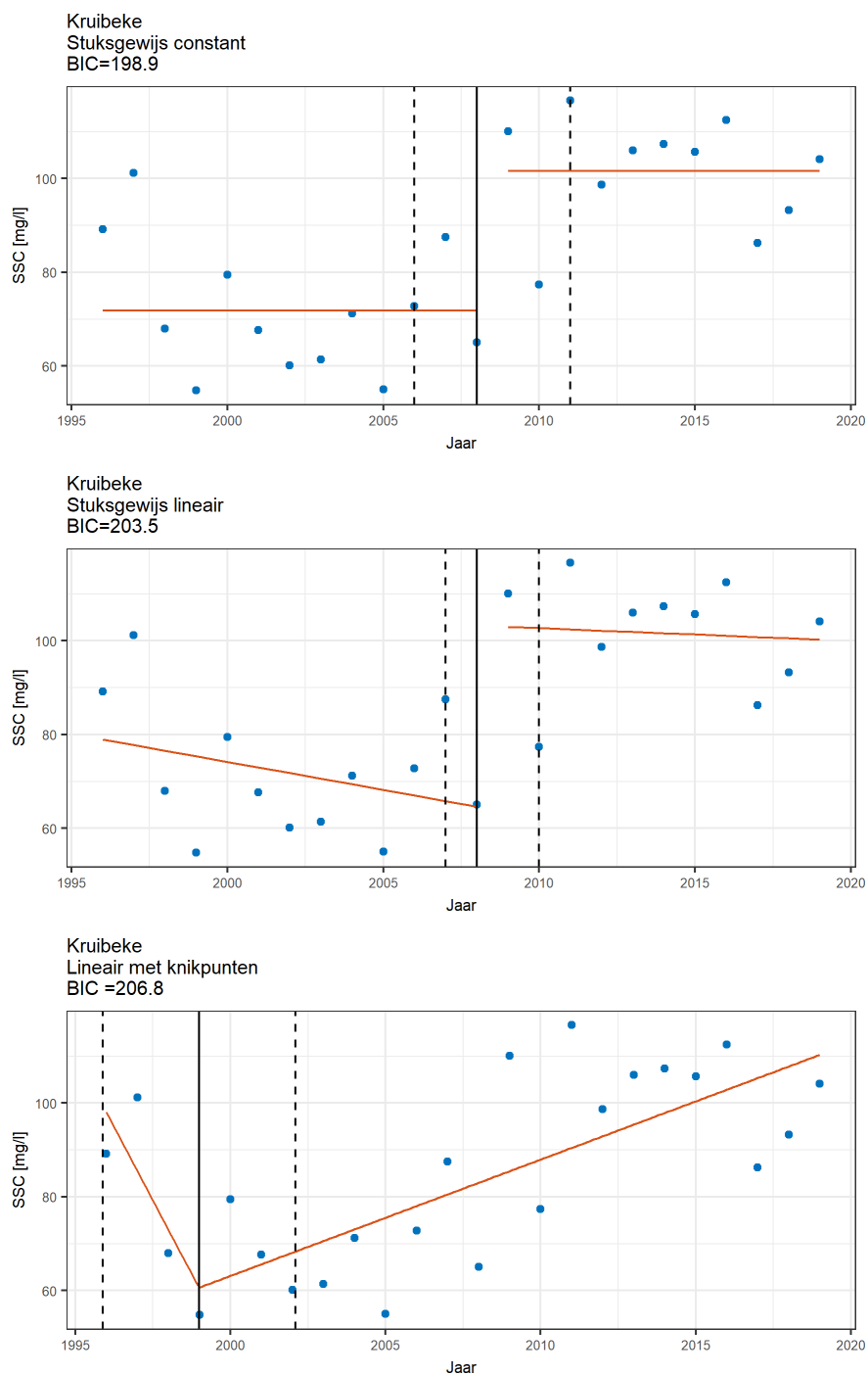
Bijlage - Figuur J-10: Drie verschillende types stuksgewijze regressie, gefit op de tijdreeks van sedimentconcentratie op meetlocatie Kruibeke. Verticale volle lijn geeft de geschatte locatie weer van de trendbreuk; verticale stippellijnen geven de 95%-betrouwbaarheidsintervallen weer.
