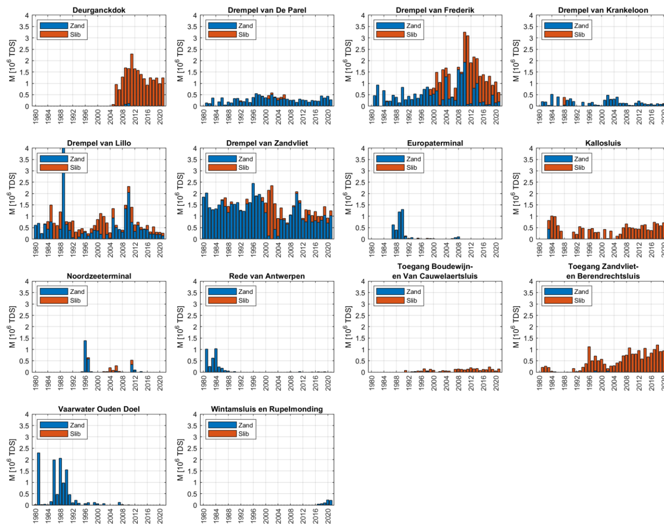
Bijlage - Figuur B-6: Totaal baggeronderhoud (zand + slib) per locatie in de Beneden-Zeeschelde (1980-2021)
