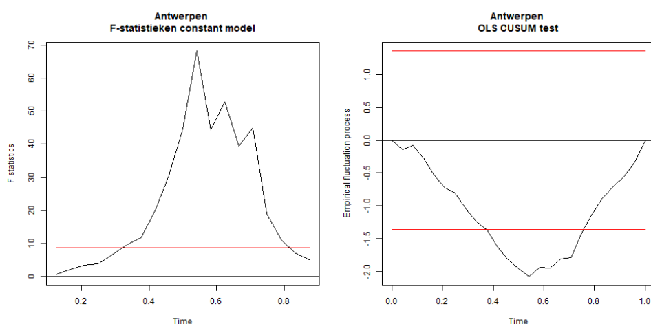
Bijlage - Figuur J-8: Controlegrafiek voor sedimentconcentratie op meetlocatie Antwerpen voor F-statistieken (links) en OLS-CUSUM (rechts).
