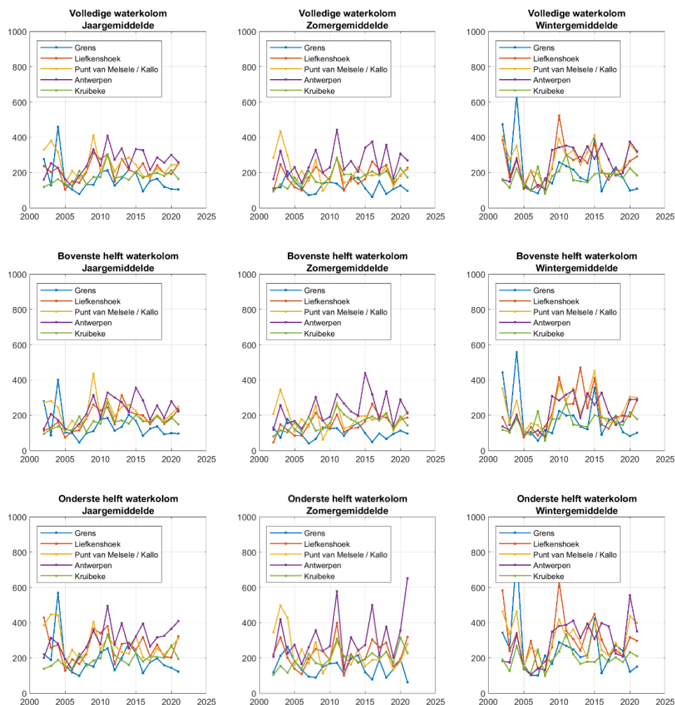
Bijlage - Figuur J-3: Sedimentconcentratie op basis van dieptestalen. Boven: volledige waterkolom. Midden: bovenste helft van de waterkolom. Onder: onderste helft van de waterkolom. Links: jaargemiddelde. Midden: zomergemiddelde. Rechts: wintergemiddelde.
