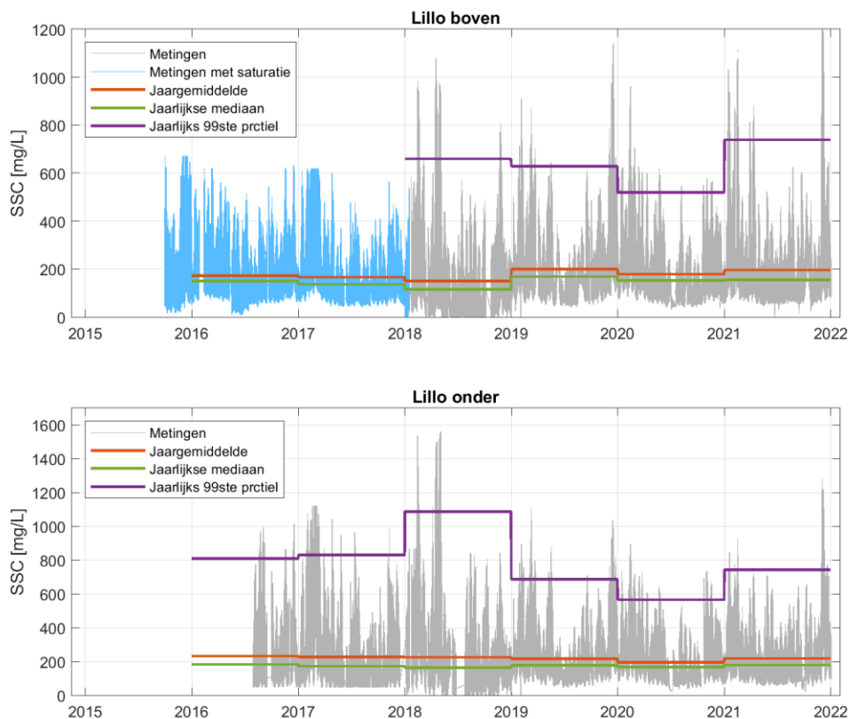
Bijlage - Figuur J-4: Continue metingen suspensiegehalte meetpaal Lillo. Metingen in blauw werden uitgevoerd met het Seaguard-500 toestel.
