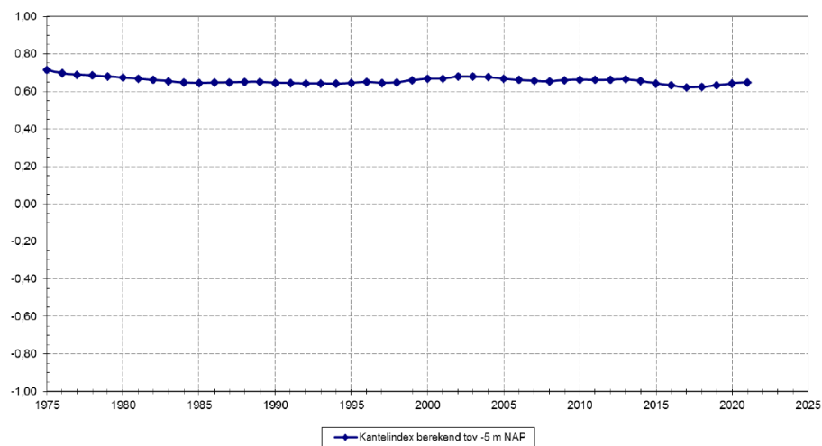
Macrocel 1 - Stabiliteit
