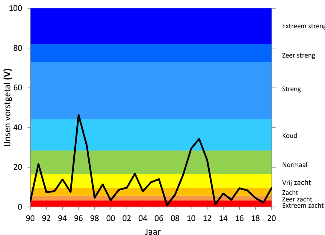
Figuur 3-1 Getal van IJsen voor de periode 1990 – 2020. De waarde voor 1990 vertegenwoordigt de winter van 1990-1991 etc.
