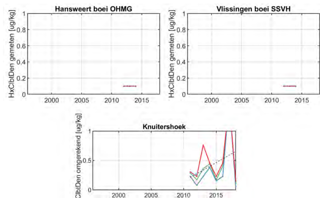
Figuur 5.28: Jaarlijks gemiddelde (groen), minimum (blauw) en maximum (rood) voor het hexachloorbutadieen in mosselen (nat en droog) voor meerdere stations. Waardes zijn in drooggewicht gepresenteerd.
