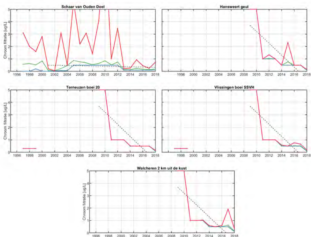
Figuur 3.67: Jaarlijks gemiddelde, minimum en maximum van het gefilterde chroomgehalte in het oppervlaktewater van de Westerschelde en de monding.
