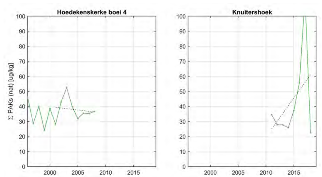
Figuur 5.22: Jaarlijks gesommeerde waarde van de 6 PAK's van Borneff in mossel bij Hoedekenskerke boei 4 en Knuitschoek. Waardes zijn in natgewicht gepresenteerd.
